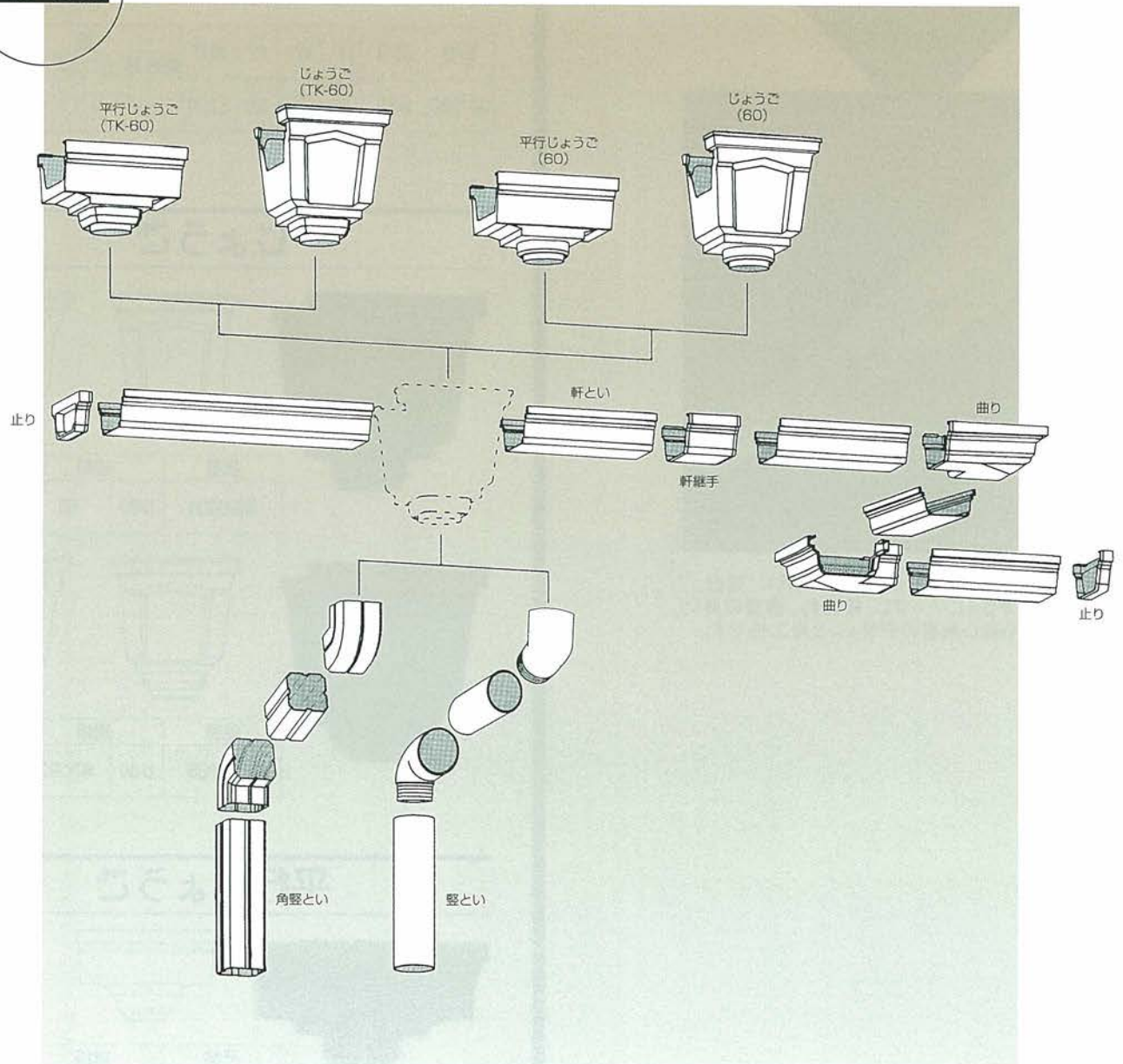
組み立て図
