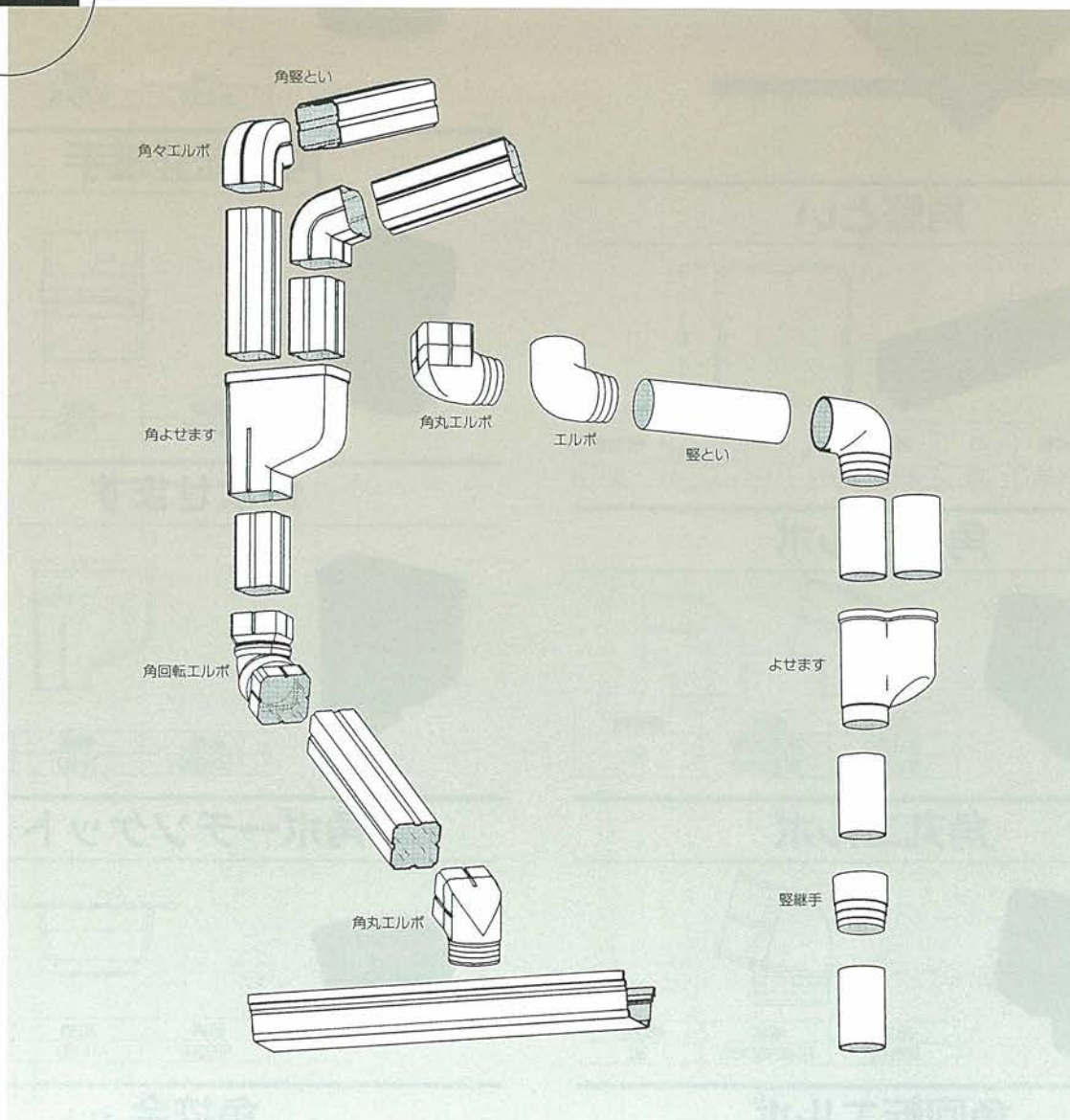
組み立て図
