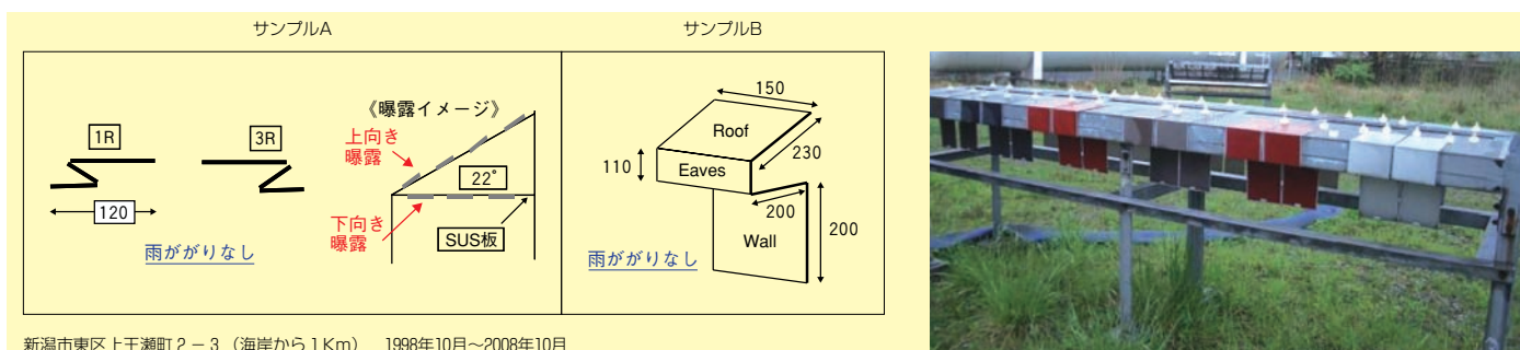
図 6-5 雨が掛からない部分のシミュレート暴露試験
