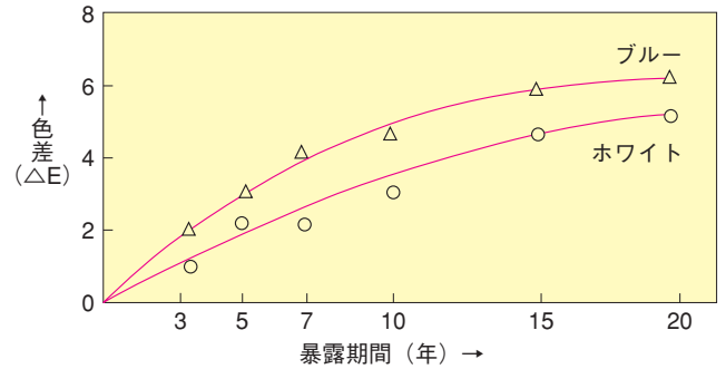
図4-4 フッ素樹脂塗装鋼板の色差の推移
