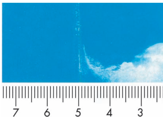
写真7-2 ふくれ 白さび
