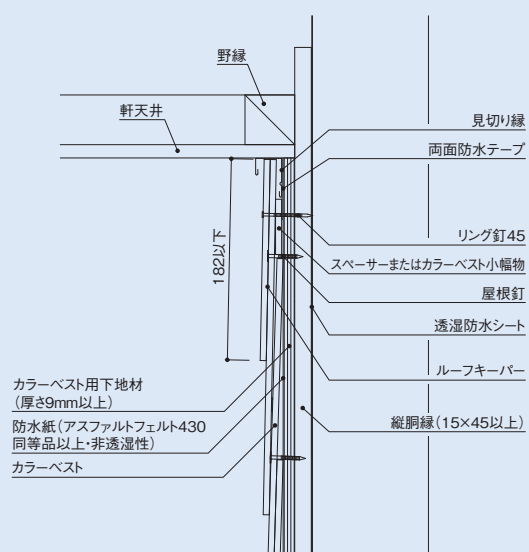
〈見切縁納まり〉
