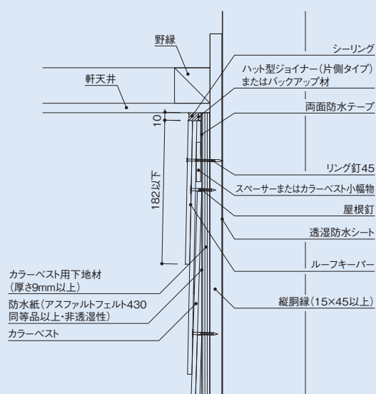
〈シーリング納まり〉
