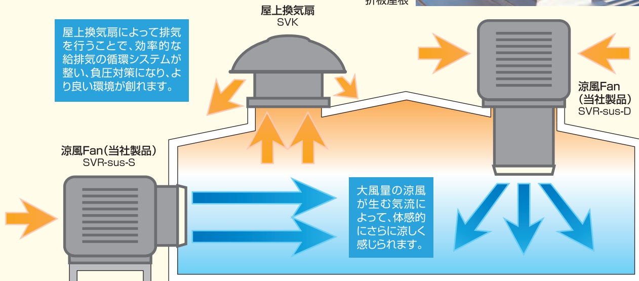
屋上取付け 折板屋根
