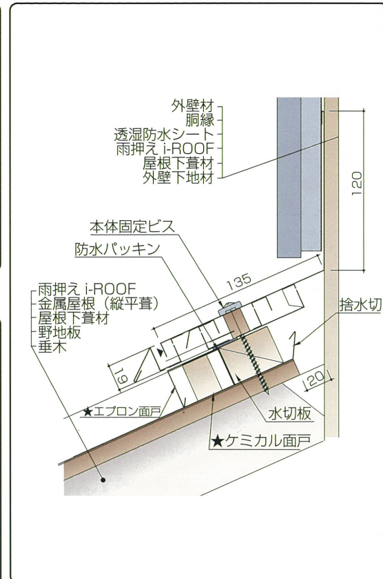
雨押え i-ROOF 施工断面図
