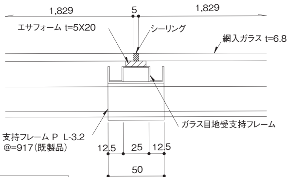
継手詳細図 1:2
