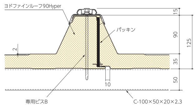
■かん合断面図
